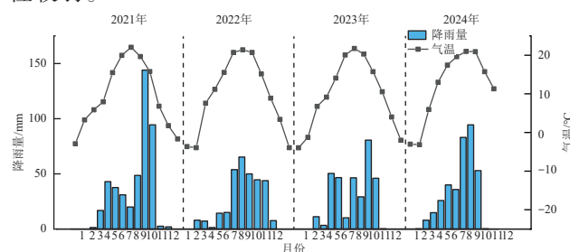
图1 2021—2024年研究区降雨量及气温变化特征
