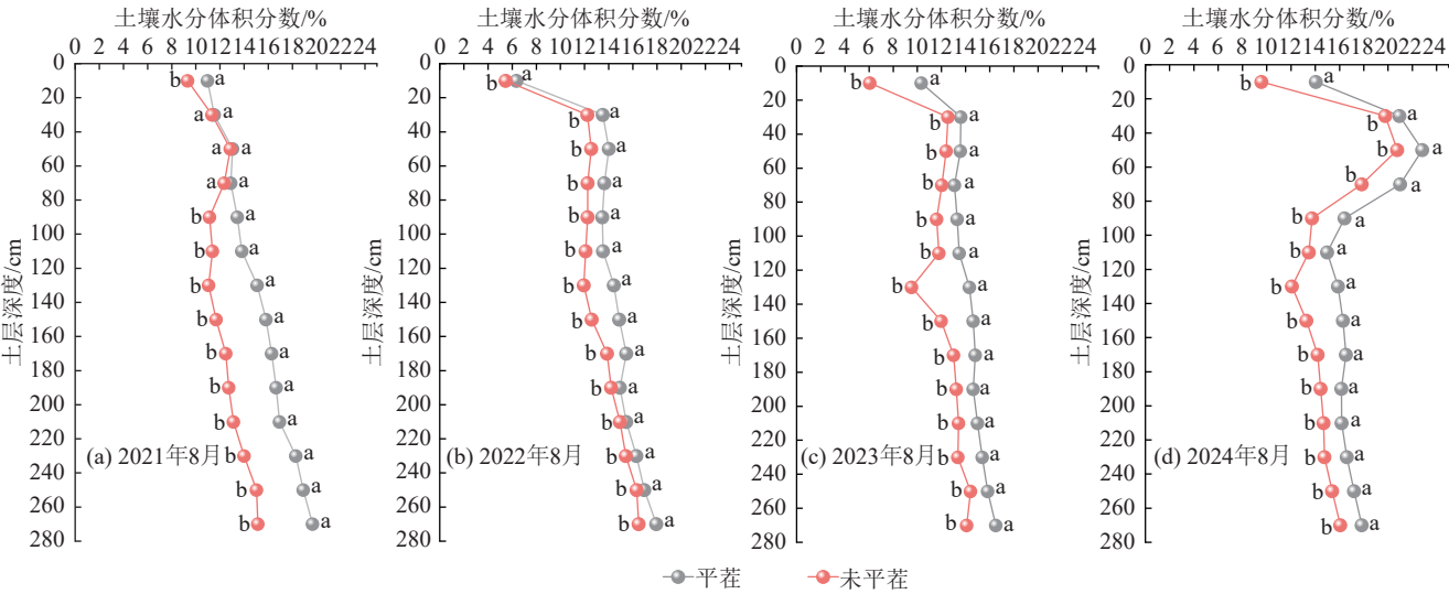
图 4 2021—2024 年 8 月土壤水分体积分数动态变化
