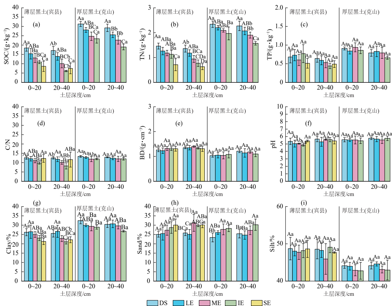
图 2 不同侵蚀强度下的土壤理化性质特征
