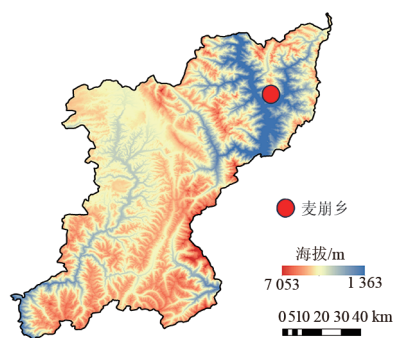
图1 研究区位置
