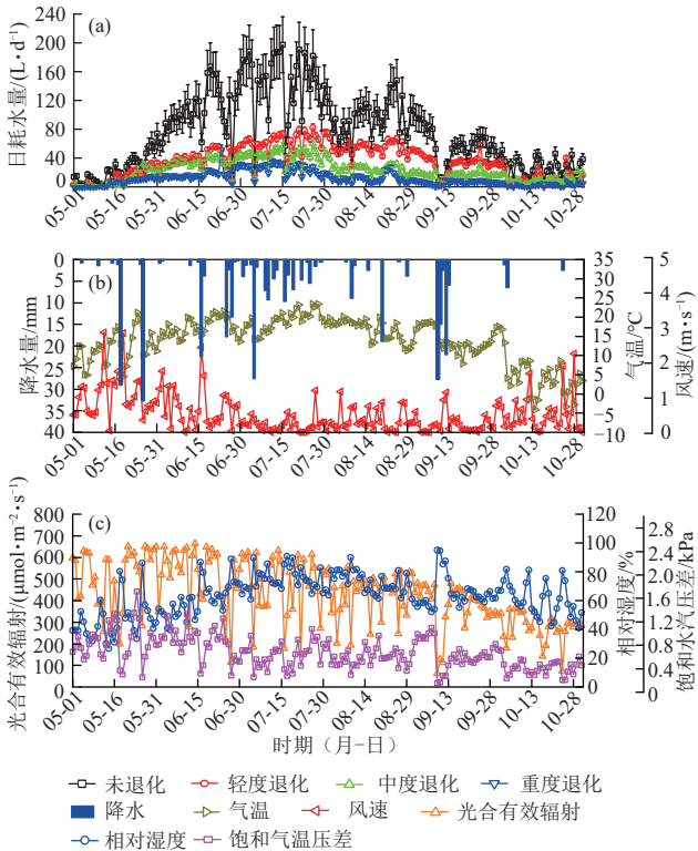
图 2 小叶杨日耗水量与气象因子时间动态变化
