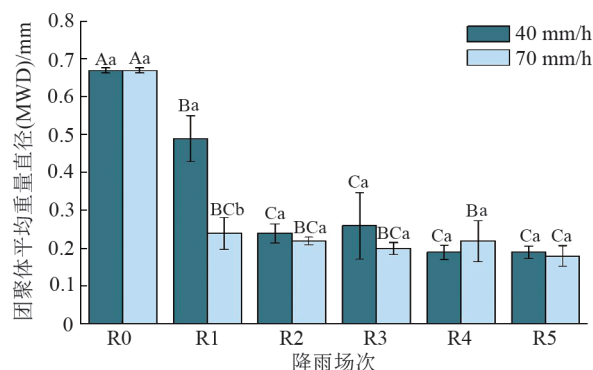
图5 不同降雨强度不同降雨次数下团聚体平均重量直径
