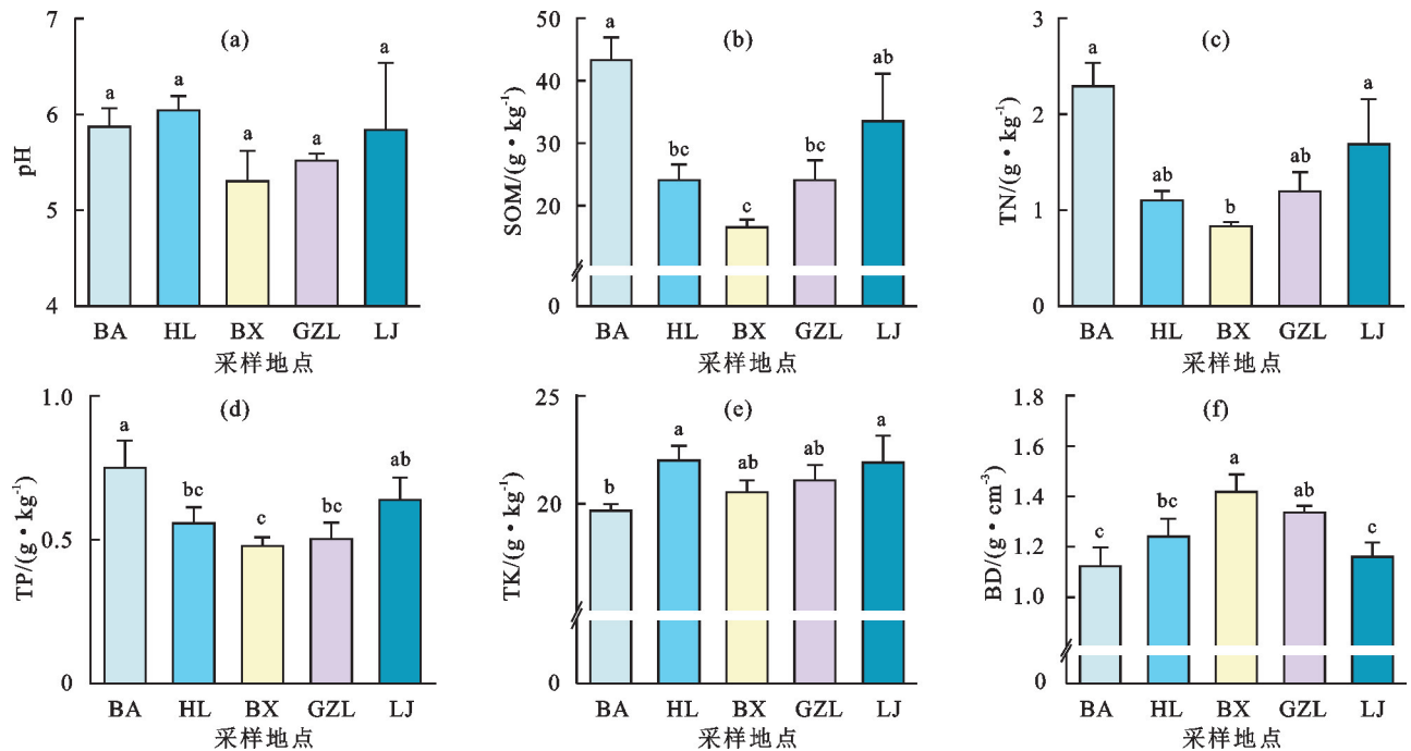
图 2 东北黑土典型水蚀区农田土壤理化性质的变化特征
