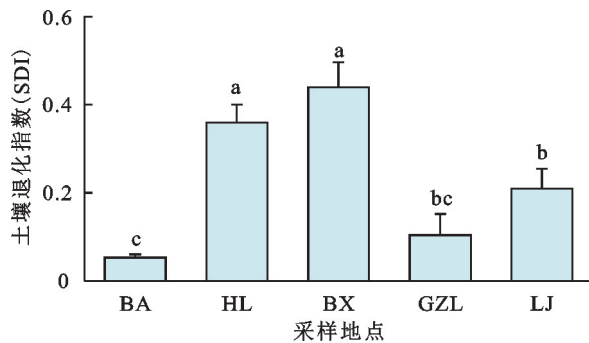
注:图柱上方不同小写字母表示地区间差异显著( p<0.05 );SDI 表示土壤退化指数(平均值±标准差)。
