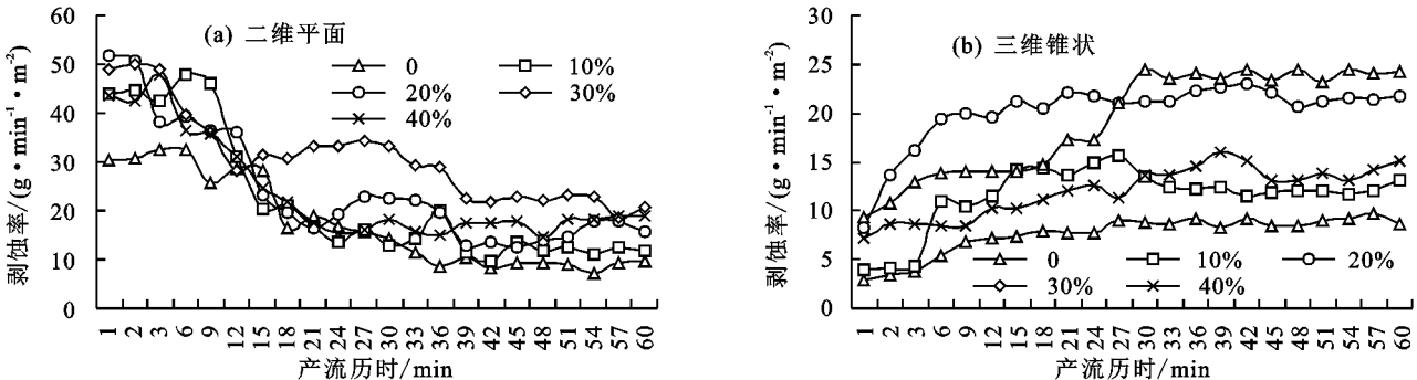
图 4 坡面剥蚀率随产流时间的变化
