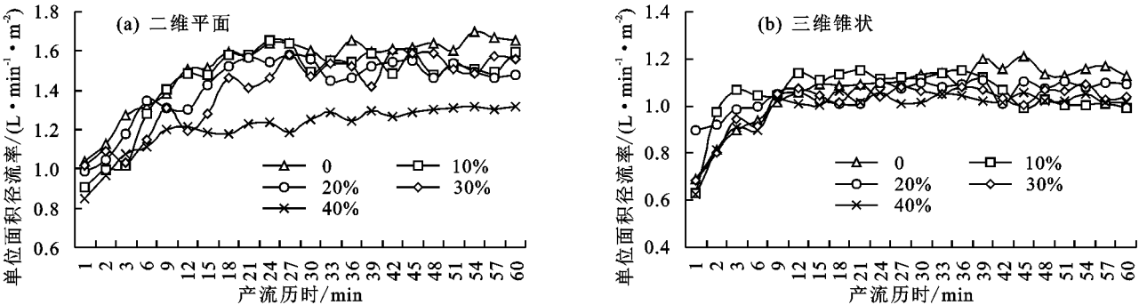
图 3 单位面积径流率随产流时间的变化
