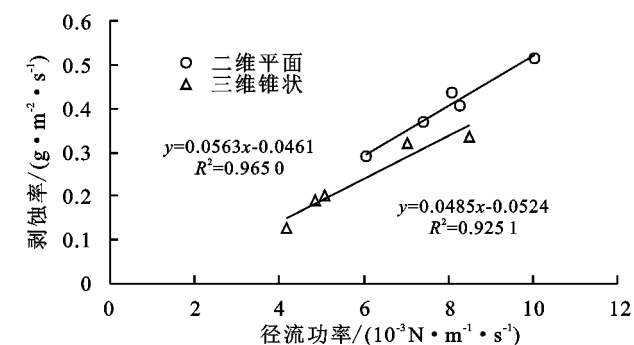
图 7 堆积体剥蚀率与径流功率的关系
