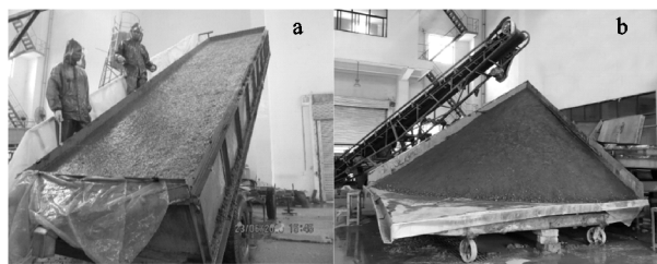
图1 二维平面堆积体坡面(a)和三维锥状堆积体坡面(b)
