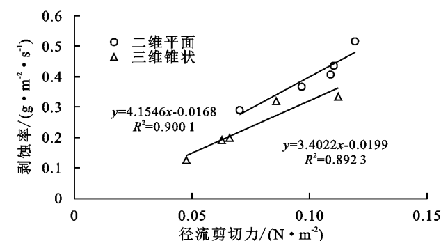
图 6 堆积体剥蚀率与径流剪切力的关系
