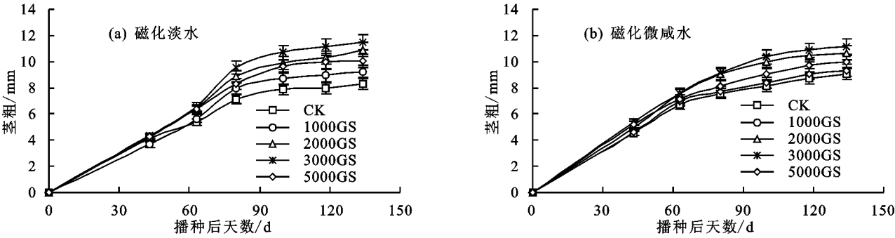
图 6 磁化水灌溉处理棉花茎粗随时间变化
