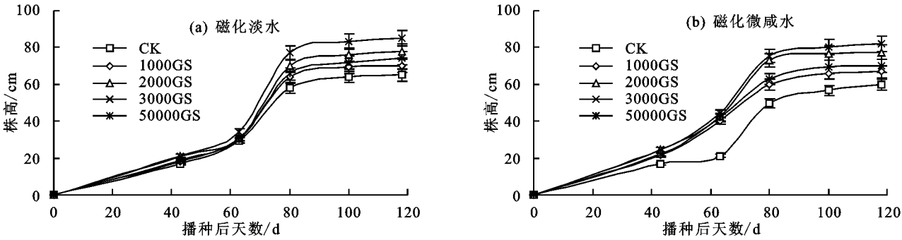
图 5 磁化水灌溉处理棉花株高随时间变化
