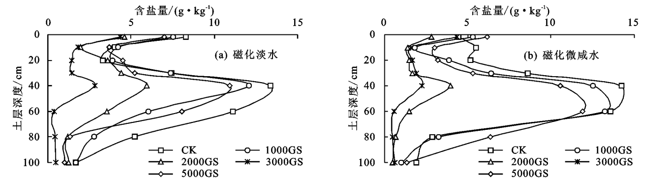
图4 磁化水灌溉处理棉花土壤盐分垂直分布
