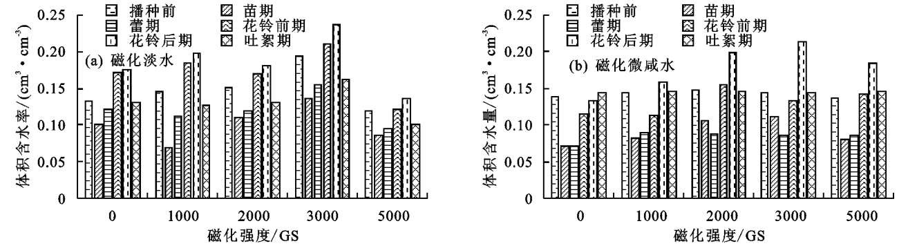
图 3 磁化水灌溉处理棉田含水量变化
