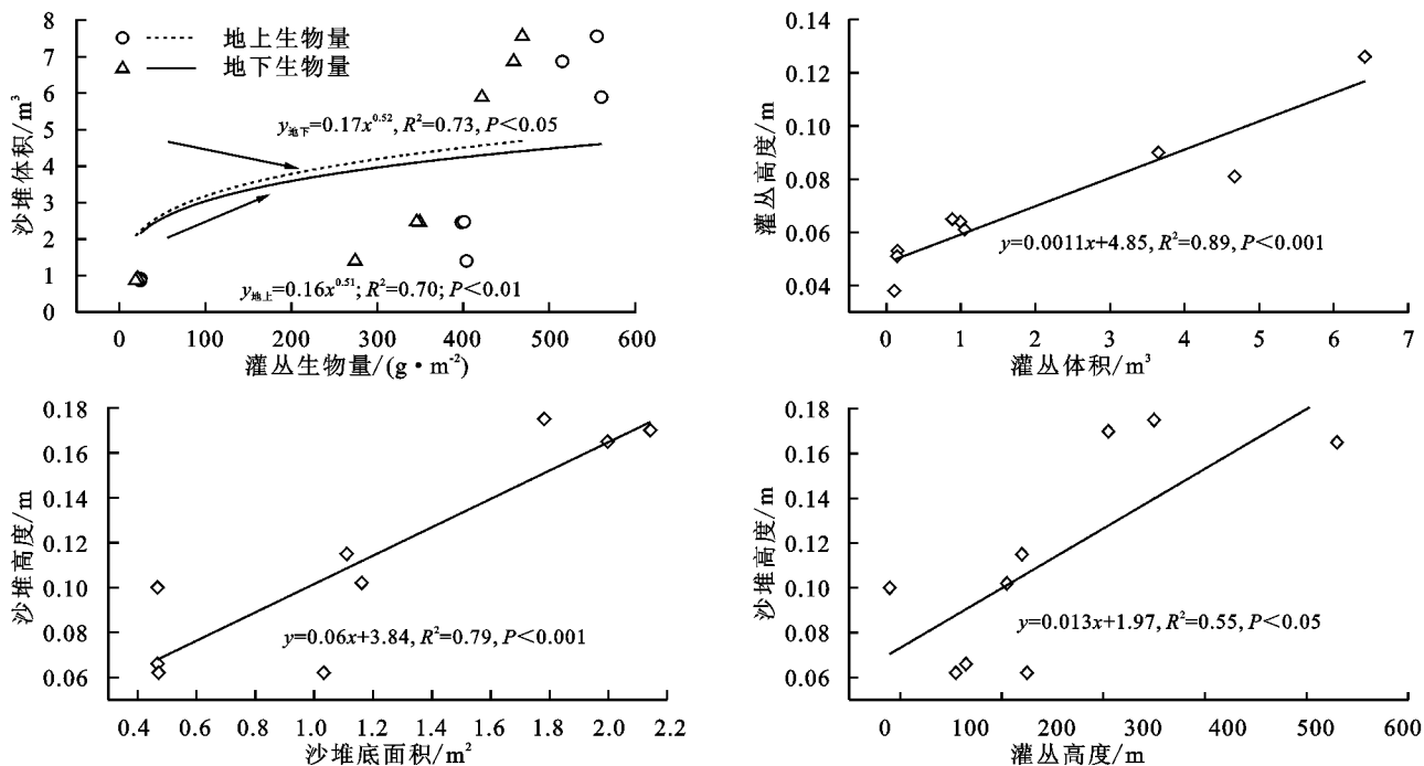
图3 灌丛生物量与沙堆体积、沙堆高度与沙堆底面积和灌丛高度、灌丛高度与灌丛体积之间关系
