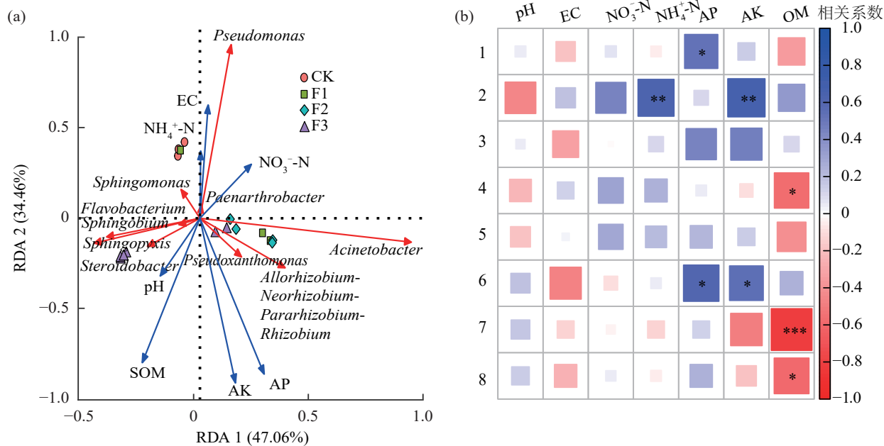
注:图a为土壤属水平群落与化学性质的RDA分析,红色箭头表示细菌属水平优势物种,蓝色箭头表示土壤化学性质;图b为细菌群落潜在碳氮循环功能与土壤化学性质的Spearman相关性热图,X轴为土壤化学性质,Y轴为细菌全磷潜在碳氮循环功能;1为芳香化合物降解,2为纤维素分解,3为芳香烃降解,4为光能异养型,5为反硝化,6为几丁质分解,7为硝酸盐还原,8为硝酸盐呼吸;色柱表示相关性,蓝色表示正相关,红色表示负相关;*表示 p<0.05 ,**表示 p<0.01 ,***表示 p<0.001 。
