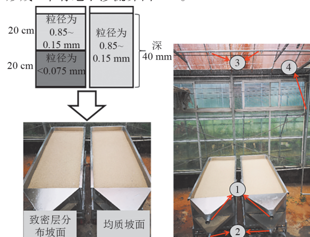
注:1为地表径流收集口;2为壤中径流收集口;3为降雨喷头;4为进水管。
