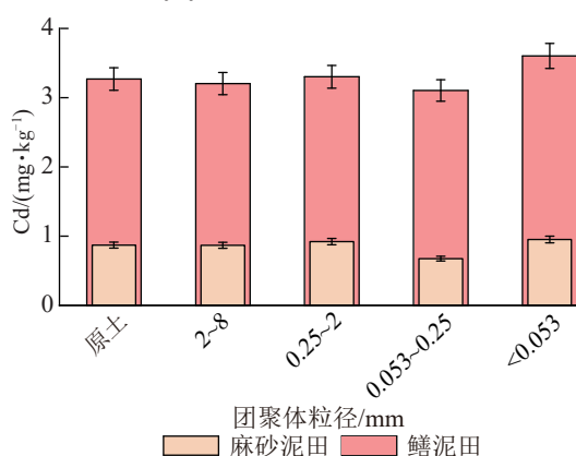
图 4 麻砂泥田与鳊泥田各粒级团聚体 Cd 质量分数
