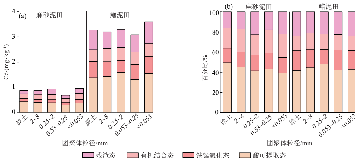
图 5 麻砂泥田与鳊泥田各粒级团聚体 Cd 形态质量分数与占比
