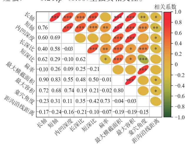
图7 龛穴形态参数相关性分析
