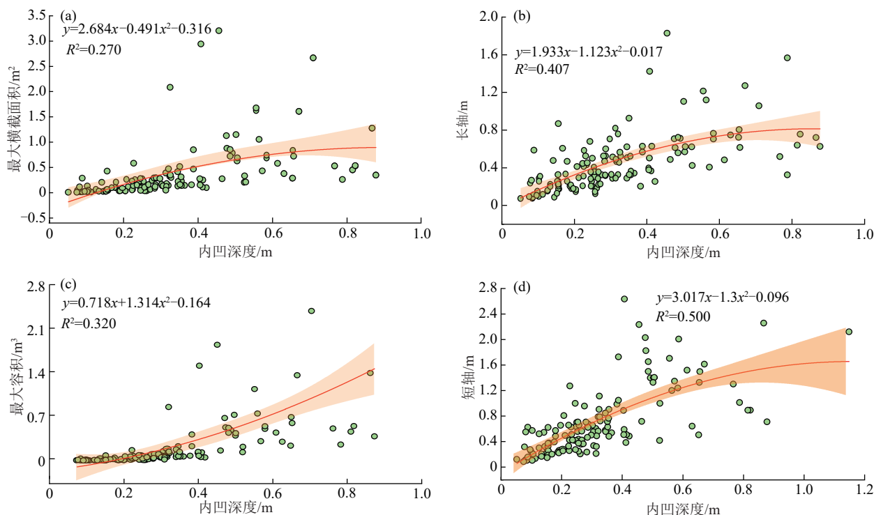
图 8 龛穴内凹深度与形态参数回归分析
