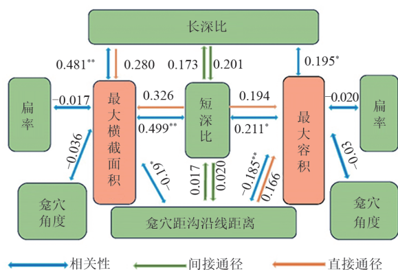
图 9 龛穴形态参数对最大横截面积、最大容积通径分析与相关性分析
