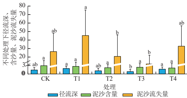
注:径流深单位为 mm,泥沙浓度单位为 kg/m³,泥沙流失量单位为 kg/hm²;图柱上方不同小写字母表示不同处理间差异显著( p<0.05 )。下同。
