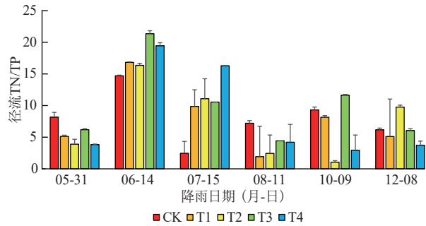
图 10 径流 TN/TP 变化 Fig. 10 Changes in runoff TN/TP ratio
