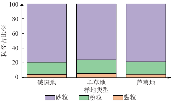
图 1 退化湿地恢复前后样地颗粒组成变化
