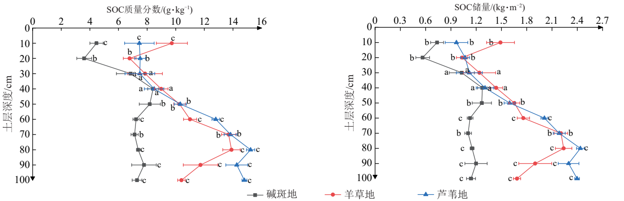
图 3 退化湿地恢复前后土壤剖面SOC质量分数与储量变化
