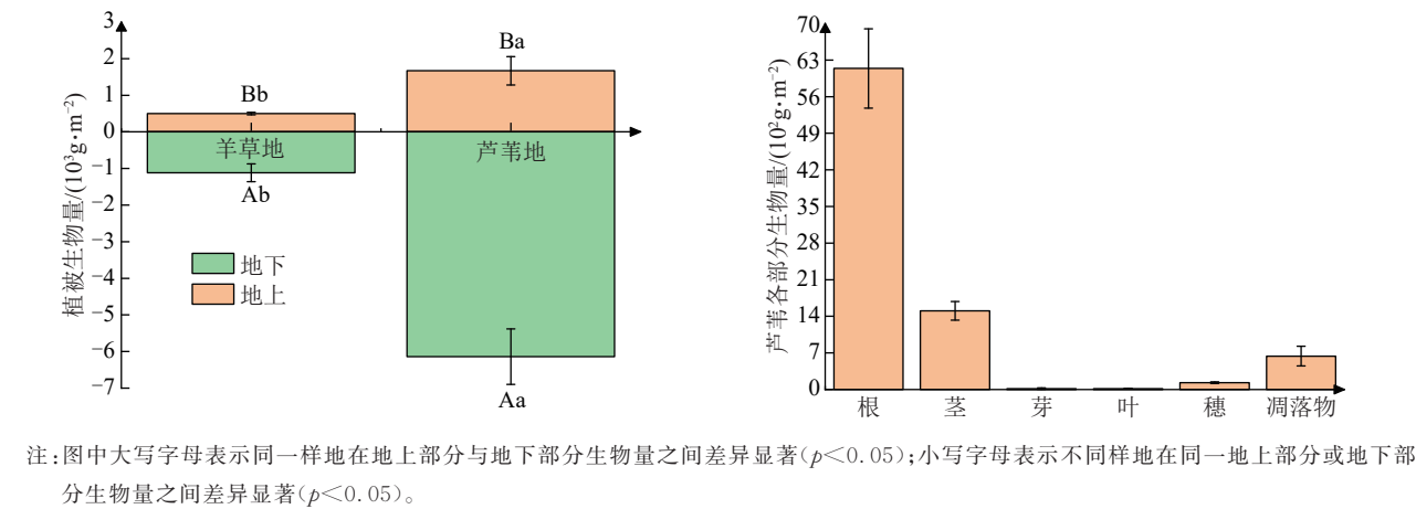
图 2 退化湿地恢复前后植被生物量变化
