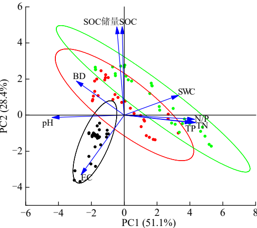
图 4 土壤有机碳含量及储量与土壤理化性质主成分分析
