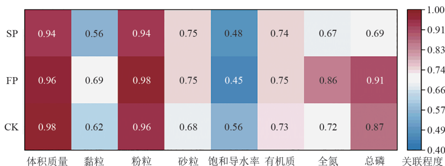
图8 不同坡耕地整地措施下土壤属性与土壤水分状况综合指数关联程度
