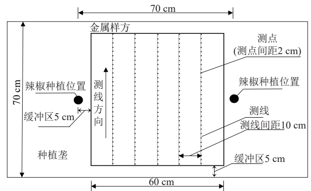
图 2 雷达探测试验测线布置与辣椒栽植示意
