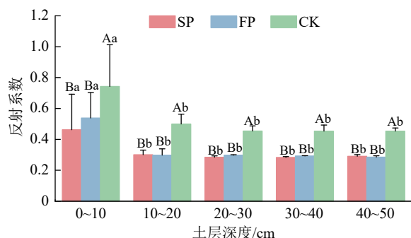
图5 不同坡耕地整地措施下田间土壤反射系数
