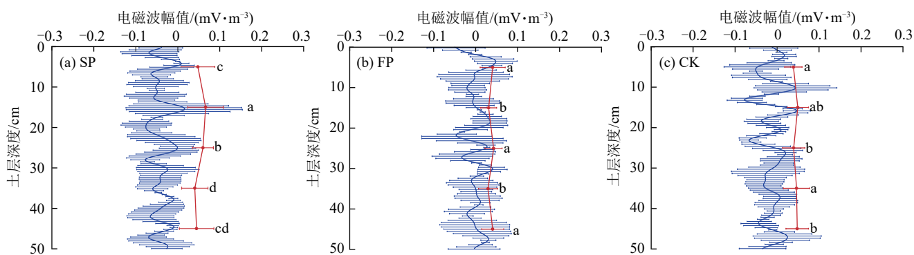
图 4 不同坡耕地整地措施下的单道波形图及其波动偏离度变化
