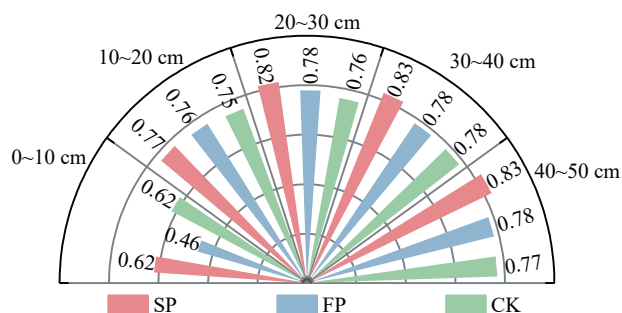
图7 不同坡耕地整地措施下供水试验前后雷达图像结构相似性指数
