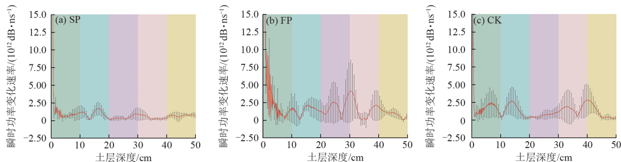
图6 不同坡耕地整地措施田间土壤瞬时功率变化速率
