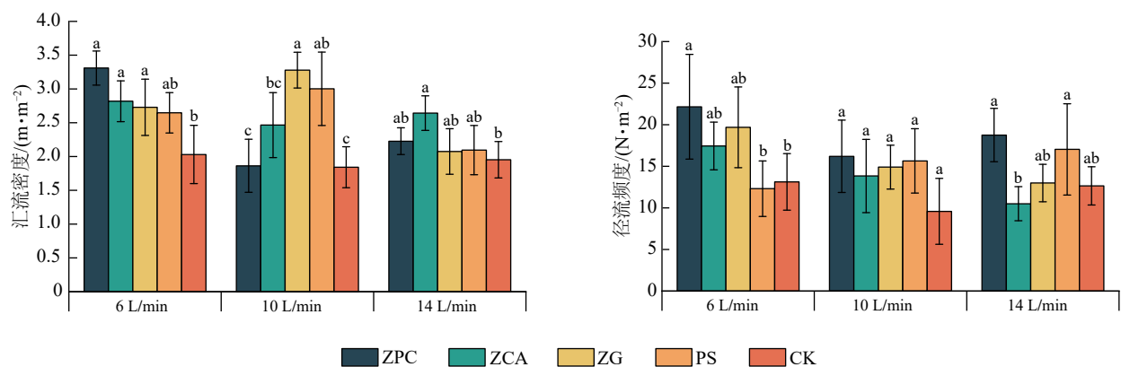
图8 汇流密度和径流频度变化特征
