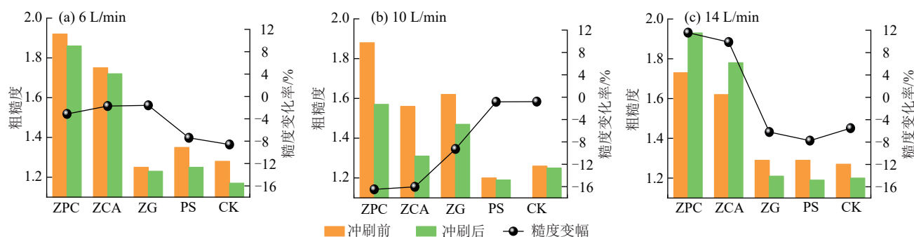
图3 不同种植模式下坡面粗糙度变化特征
