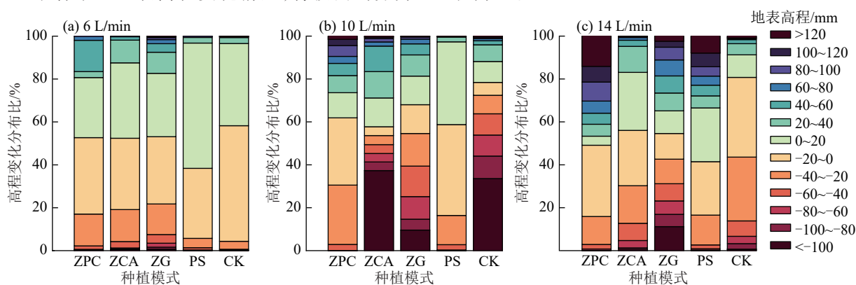
图2 不同种植模式下微地形高程量变化量分布比例
