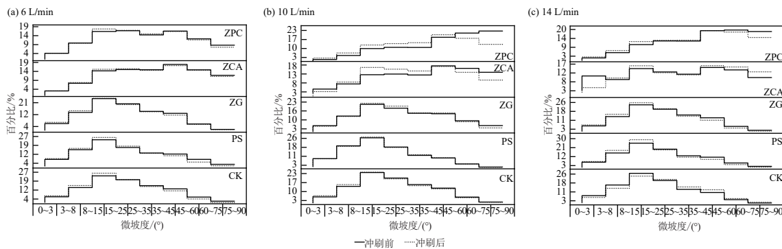
图 5 微坡度分布特征
