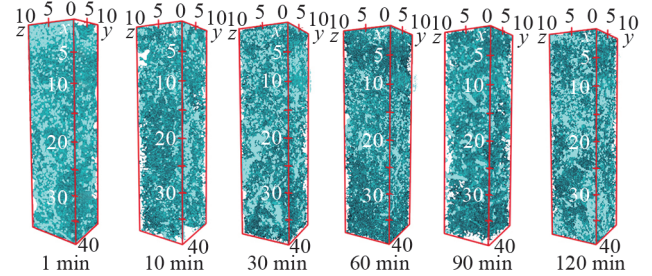
注:柱形图中的 x 轴为纵轴,向下指示土层深度; y 、 z 轴为平面切片,表示裁剪出的 10 \text{ mm} \times 10 \text{ mm} 的正方形感兴趣区域。
