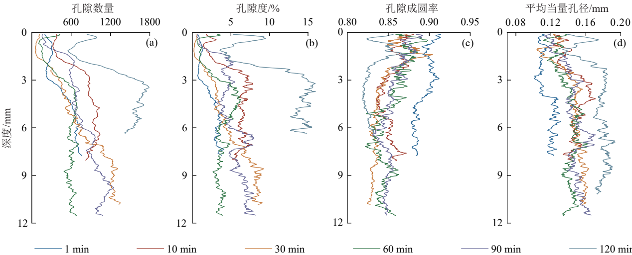
图 4 结皮土样二维指标垂直分布特征
