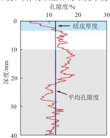
图1 结皮厚度量化示意
