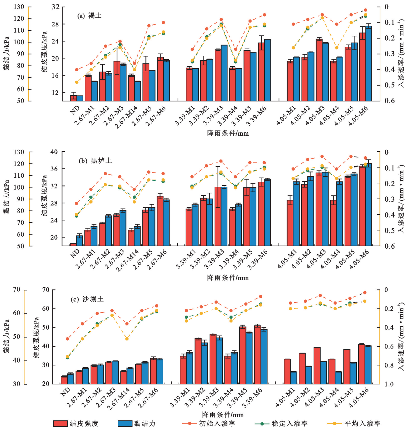
图 2 不同降雨条件下形成的结皮与入渗性能的关系
