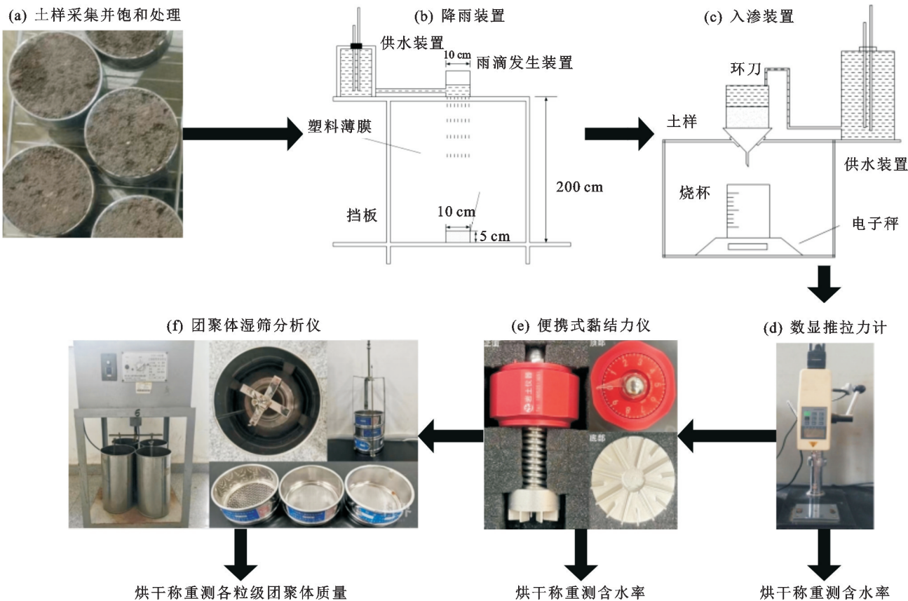
图 1 试验装置及流程
