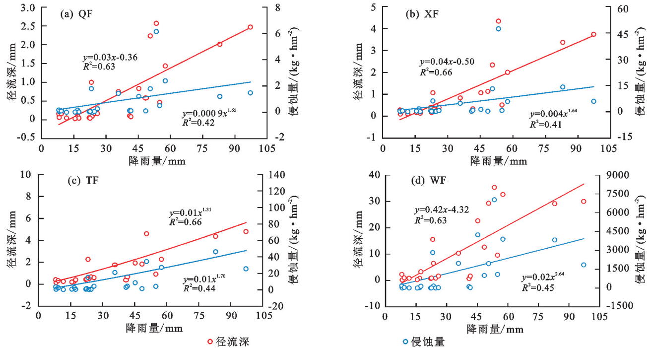
图 6 不同林草覆被格局降雨量与侵蚀量、径流量的关系
